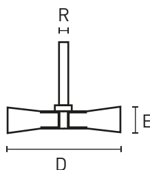
Microcepillo con eje
